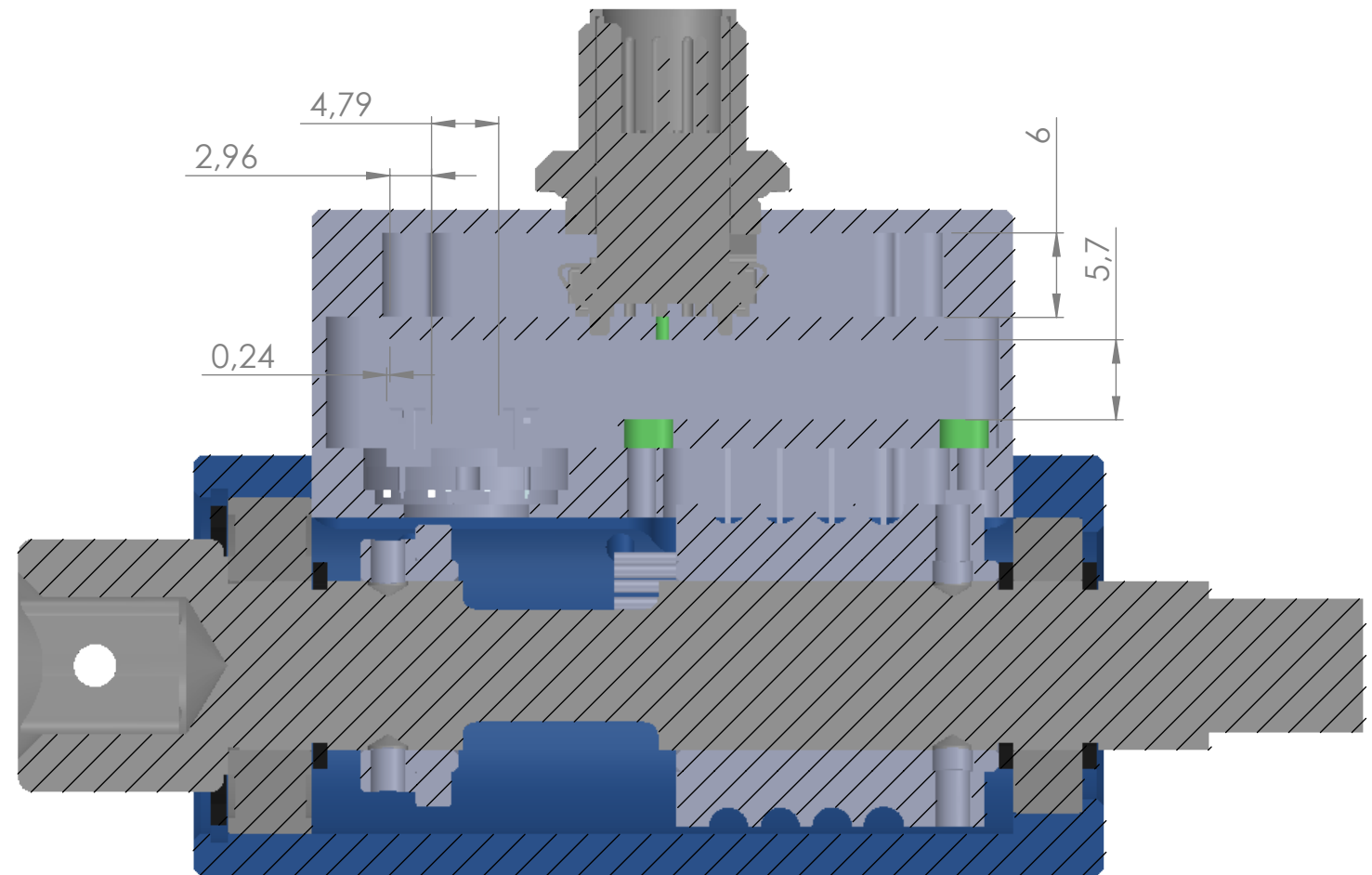
SEZIONE B-B SCALA 2 : 1
